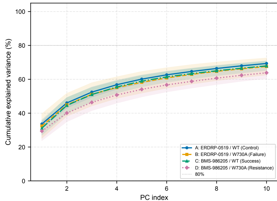
PCA — global
